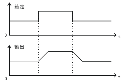
图 2-10 阶跃给定下输出的变化
