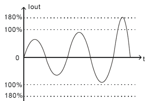
图 2-8 过流保护特性
