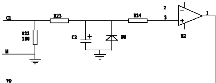
图6-1 4~20mA转换回路
