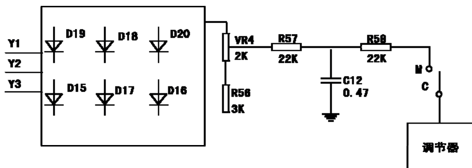
图6-3 电压反馈取样电路
