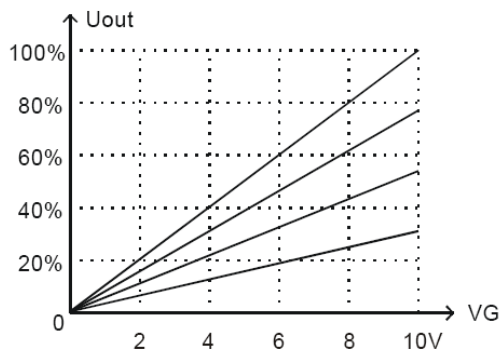
图2-2 “斜率”调节特性
