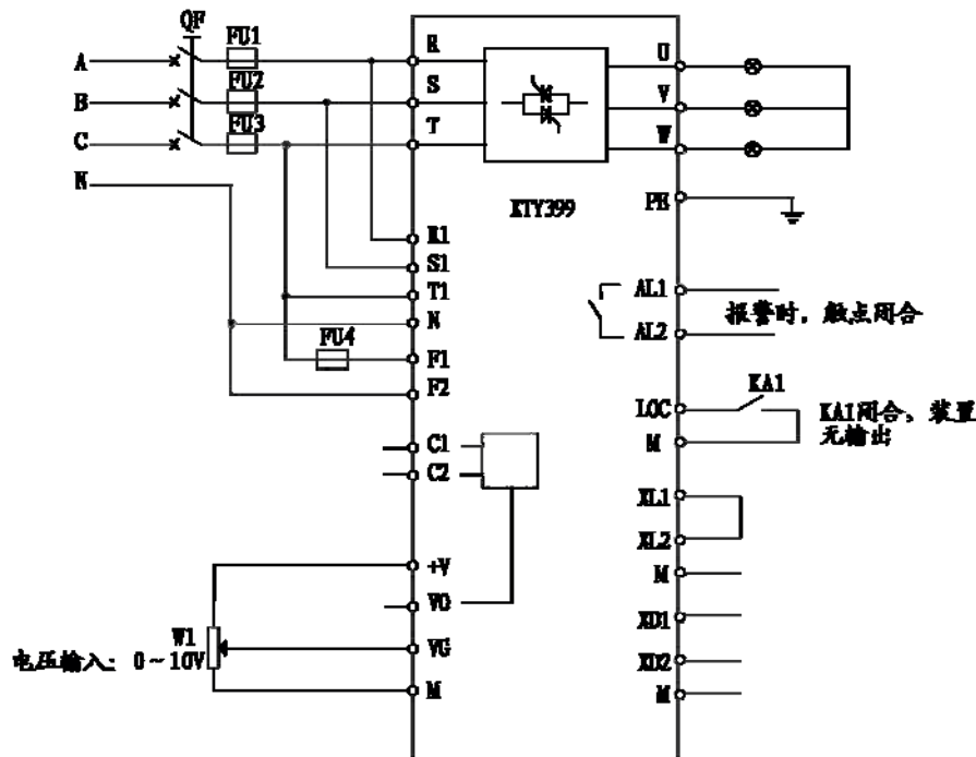
图5-1 试验接线
